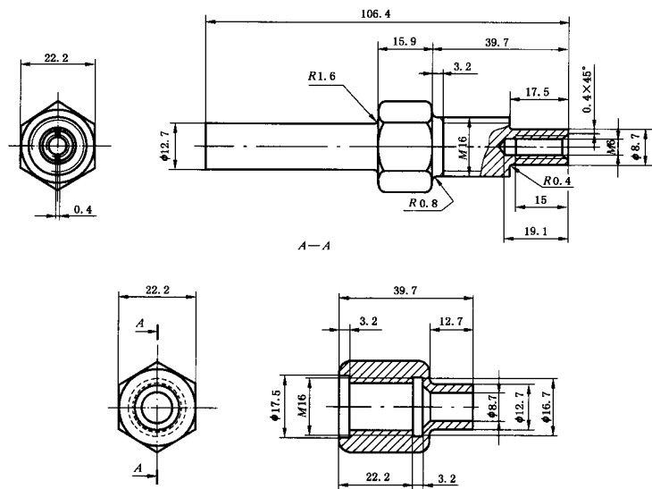
图4 抛光试棒用的夹头
