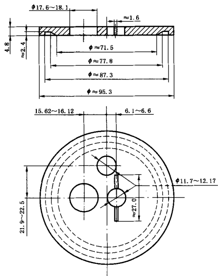
图 2 烧杯盖
